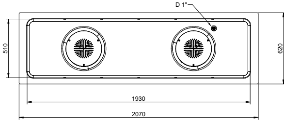
Üst
