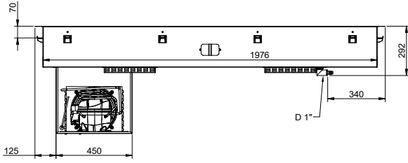
Arka taraf
